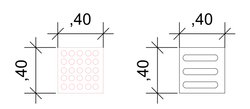
PISO PODOTÁTIL ESC. S/ESC
