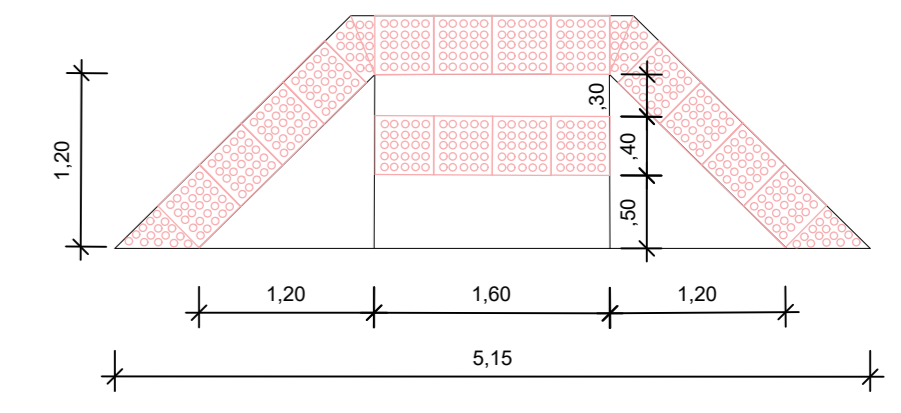
RAMPAS DE ACESSIBILIDADE ESC. 1/50
