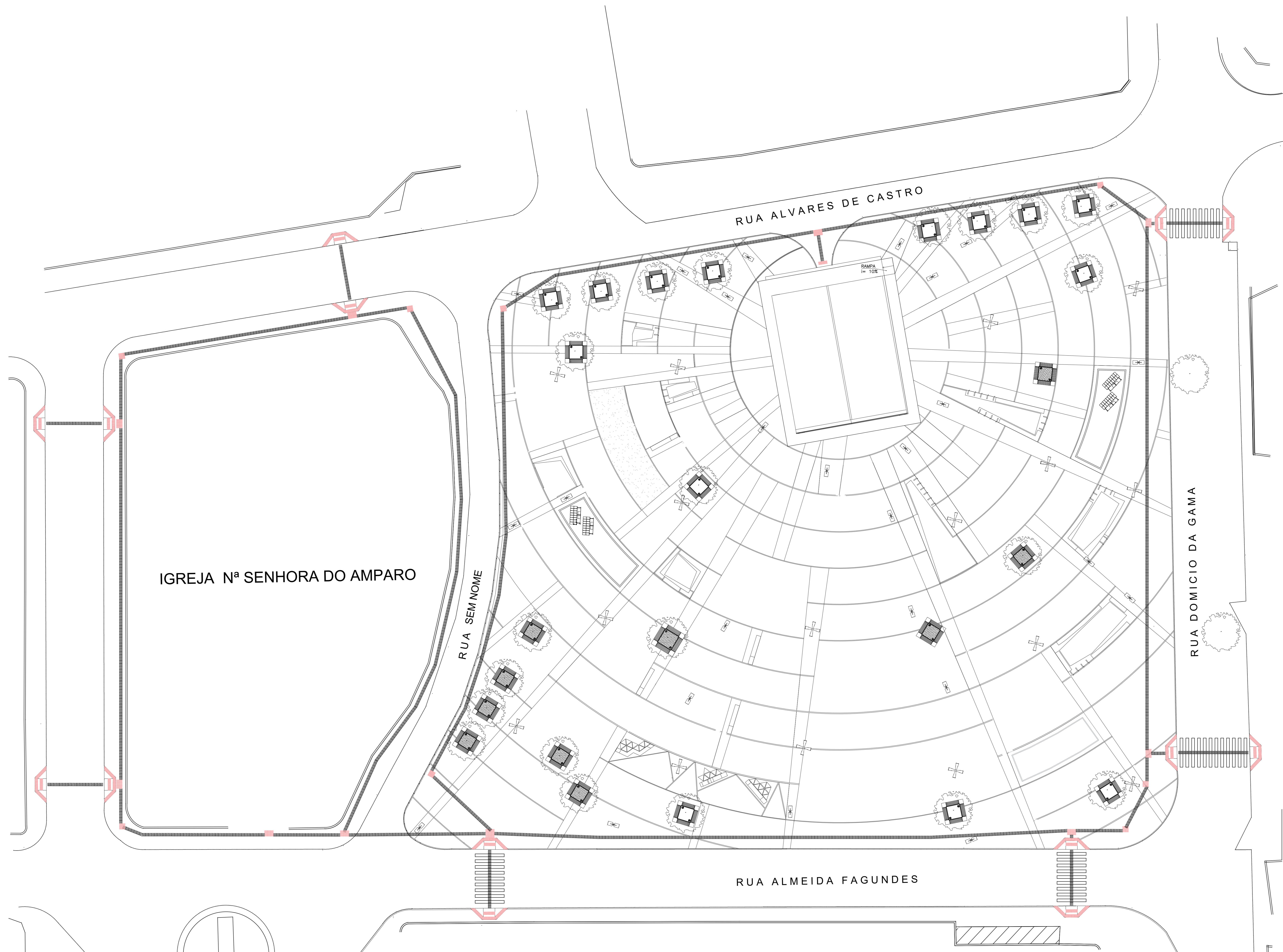
RAMPAS DE ACESSIBILIDADE ESC. 1/50
