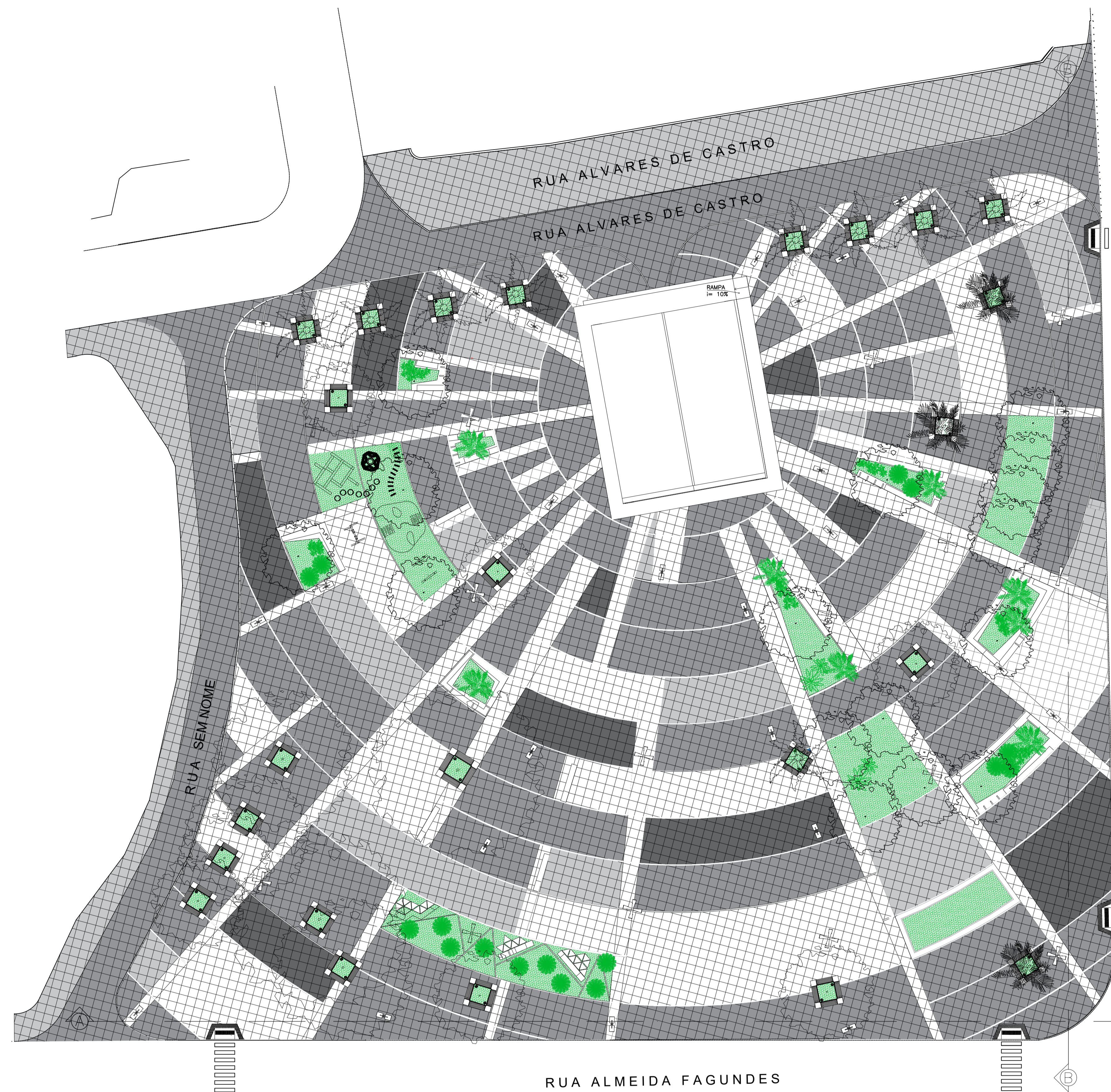
01 PLANTA DE IMPLANTAÇÃO ESC. 1/200
